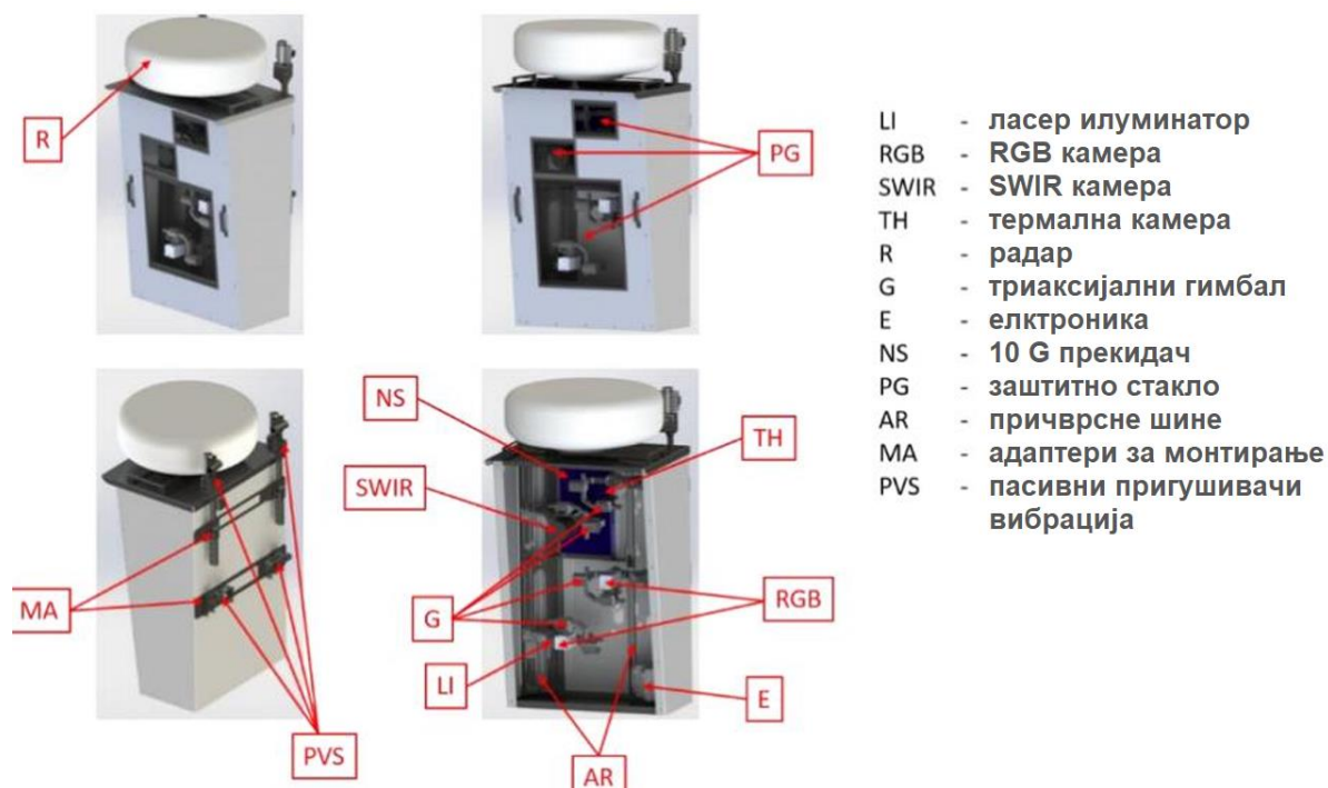
Слика 8.3 CAD модел интегрисаног система OD&TID на челу локомотиве [88]
